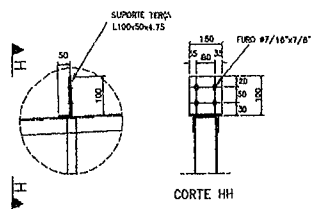
DET. 01(SUPORE TERÇA)
