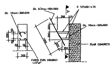
SUPORE DAS CALHAS
