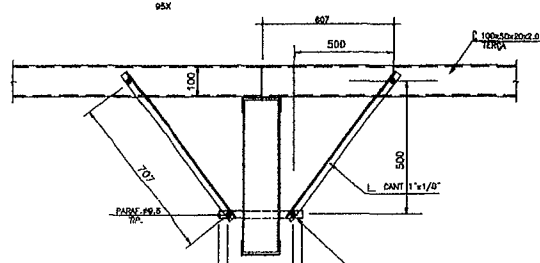
DETALHE MÃO FRANCESA
