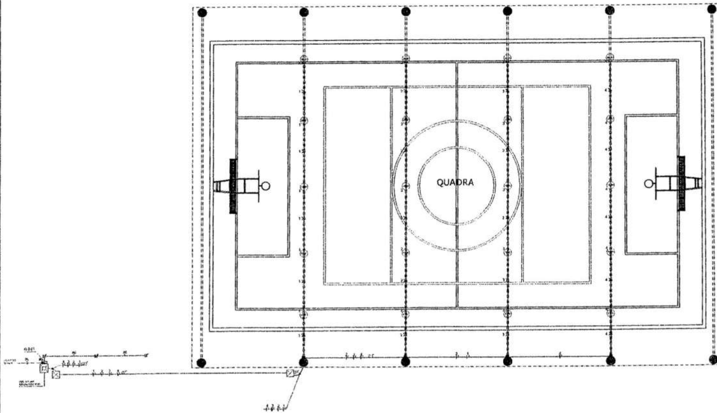
1 PLANTA DE ELÉTRICO ESCALA 1/75
