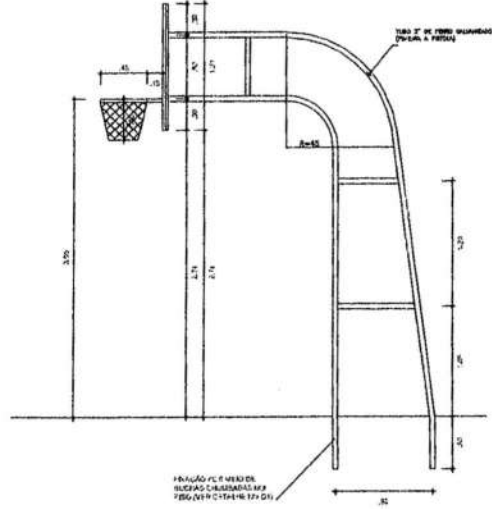
1 DETALHE TABELA DE BASQUETEBOL ESCALA 1/25
