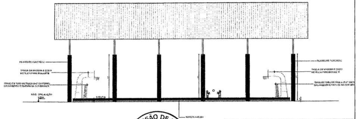
2 VISTA 02 QUADRA ESCALA 1/100
