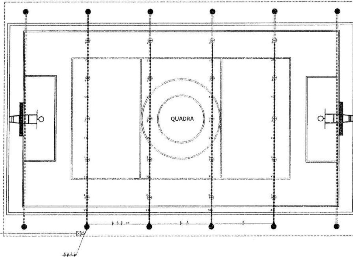
1 PLANTA DE ELÉTRICO ESCALA 1/75
