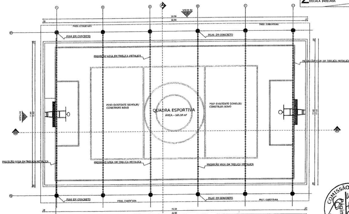
1 PLANTA DE BAIXA ESCALA 1/75
