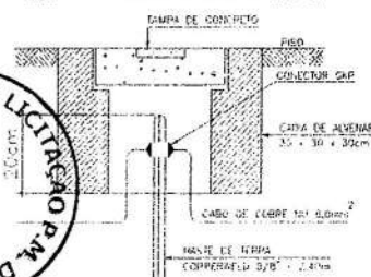
DETALHE ATERRAMENTO
