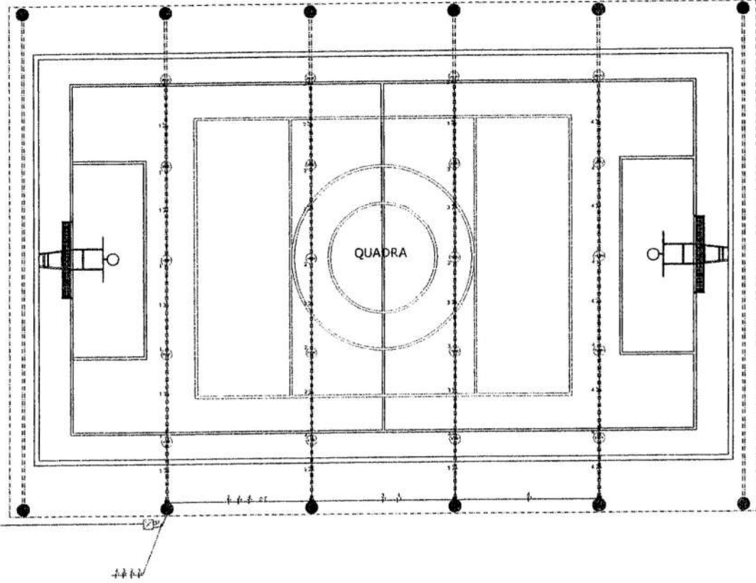
1 PLANTA DE ELÉTRICO ESCALA 1/75
