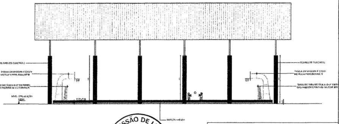
2 VISTA D2 QUADRA ESCALA 1/100
