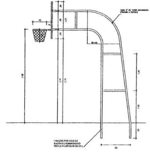
1 DETALHE TABELA DE BASQUETEBOL ESCALA 1/25
