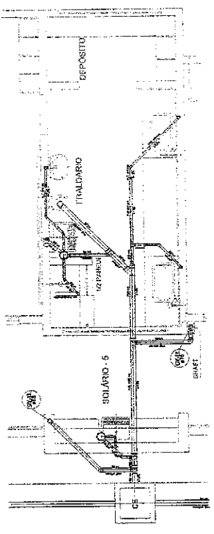
Detalhe S10 escala 1:25
