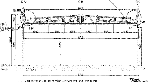
6 BLOCO C - ELEVACÃO - EXO C3, C4, C5 E C6 ESCALA: 1/50
