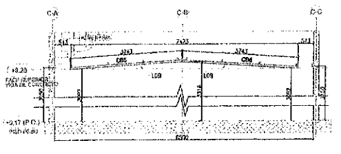
2 BLOCO C - ELEVACÃO - EXO C1 E C2 ESCALA: 1/50
