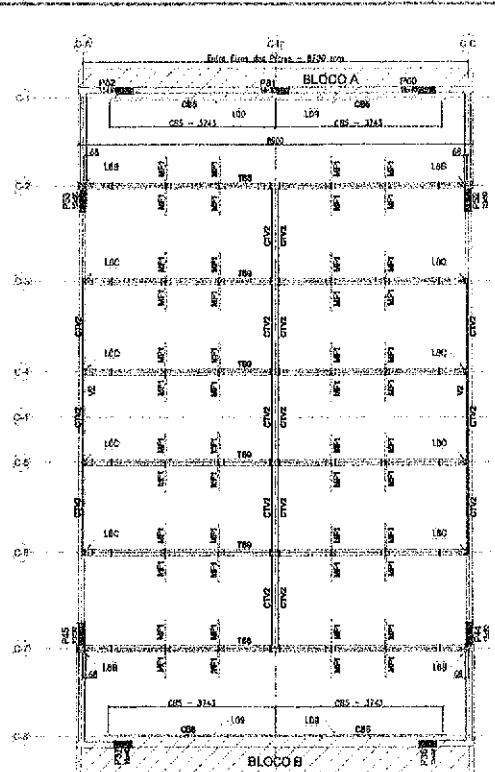
4 BLOCO C - VISTA EM PLANTA - VIGAS, TESOURAS, CAIBROS E MÃOS-FRANÇÊSAS ESCALA: 1/50
