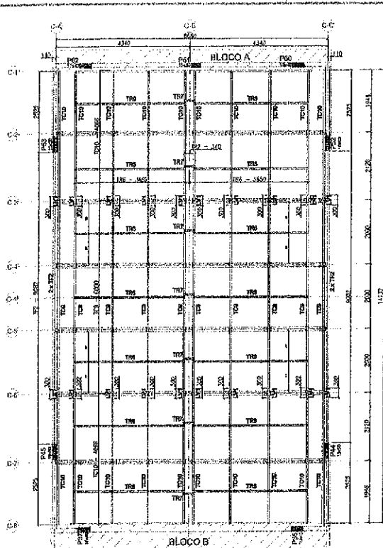
1 BLOCO C - PLANTA DE COBERTURA - TESOURAS, TERÇAS, TRAVAMENTOS e CAIBROS ESCALA: 1/50
