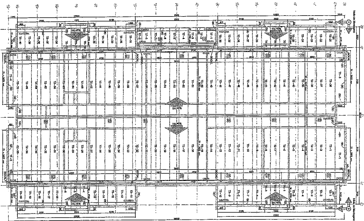
1 BLOCO B - PLANTA DE COBERTURA ESCALA: 1/50
