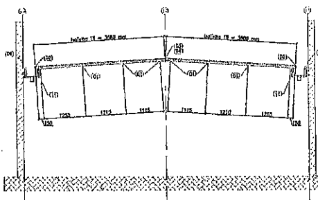
3 BLOCO C - ELEVACÃO - EIXO C2 E C7 ESCALA: 1:50
