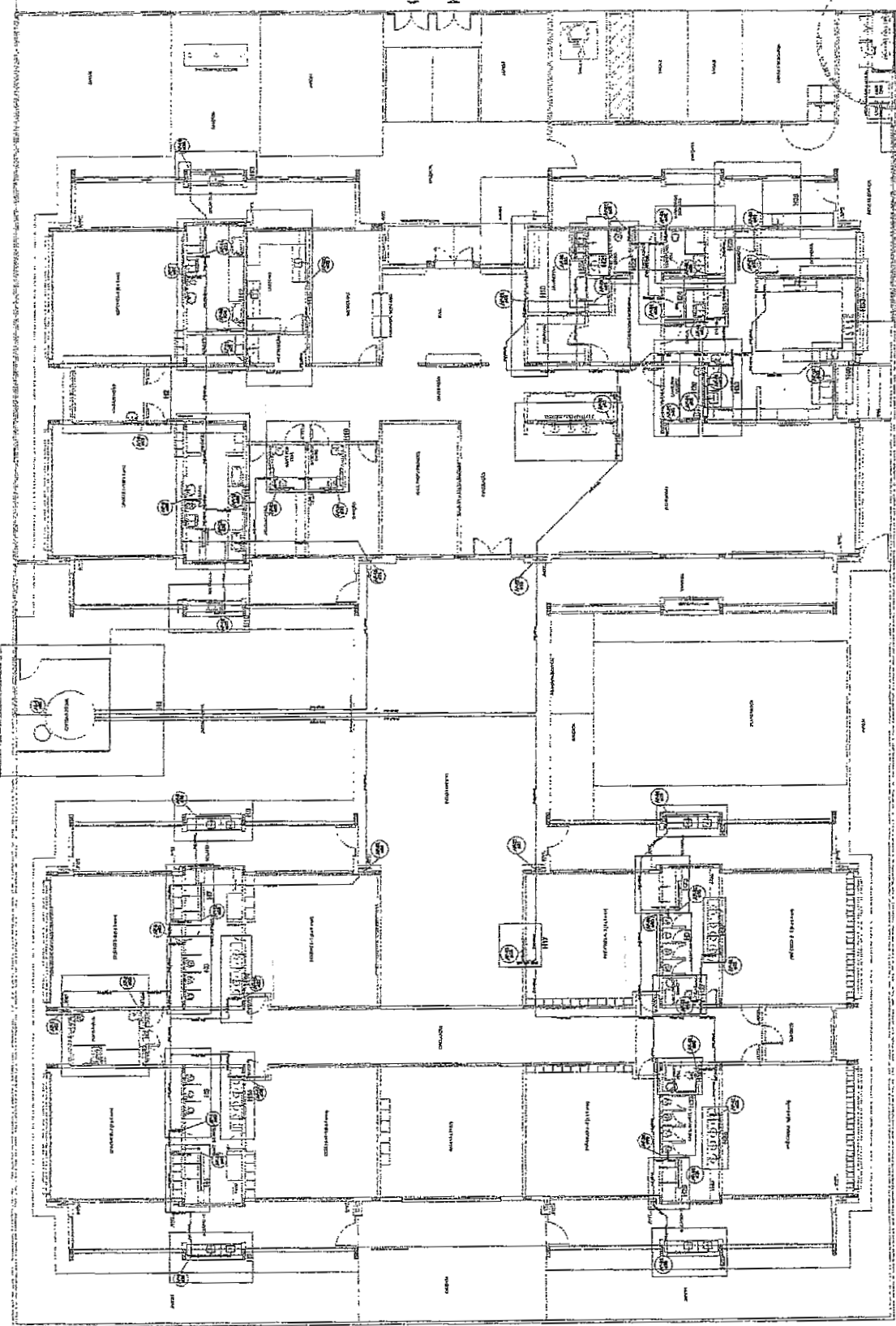
PLANTA GERAL
