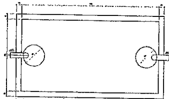
TANQUE SÉPTICO PLANTA BAIXA - ESC. 1:25
