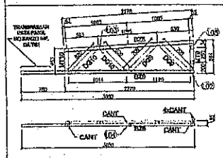
VISTA SUPERIOR - BANZOS, CANTONEIRAS e LUVAS
