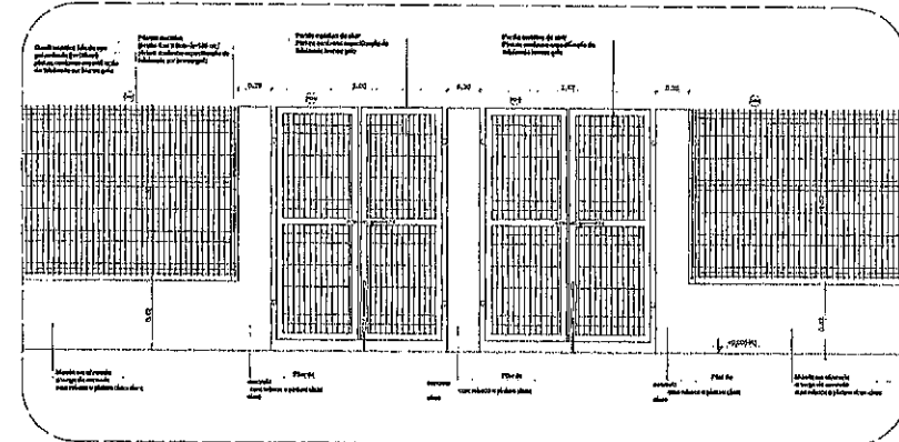
6 AMPLIAÇÃO - PORTÃO DE ACESSO E GRADIL DE FECHAMENTO FRONTAL ESCALA 1/20
